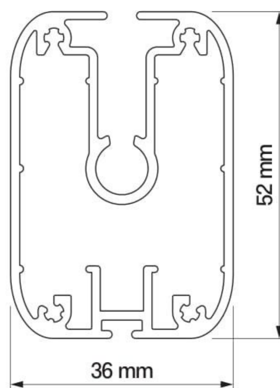
Fallprofil FG51
