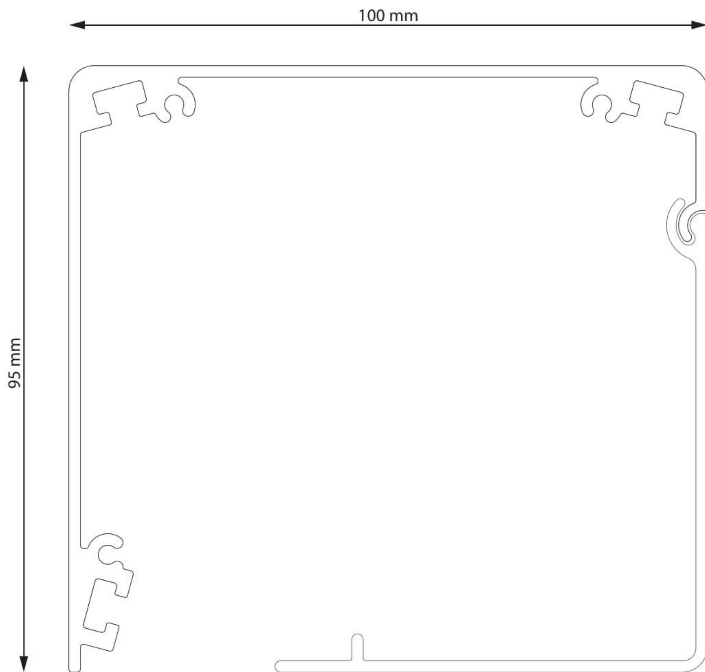
ZiiiP 95 Querschnitt der Kassette
