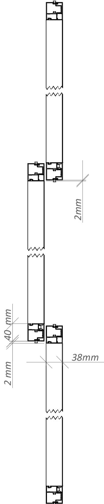
GRUNDRISS
