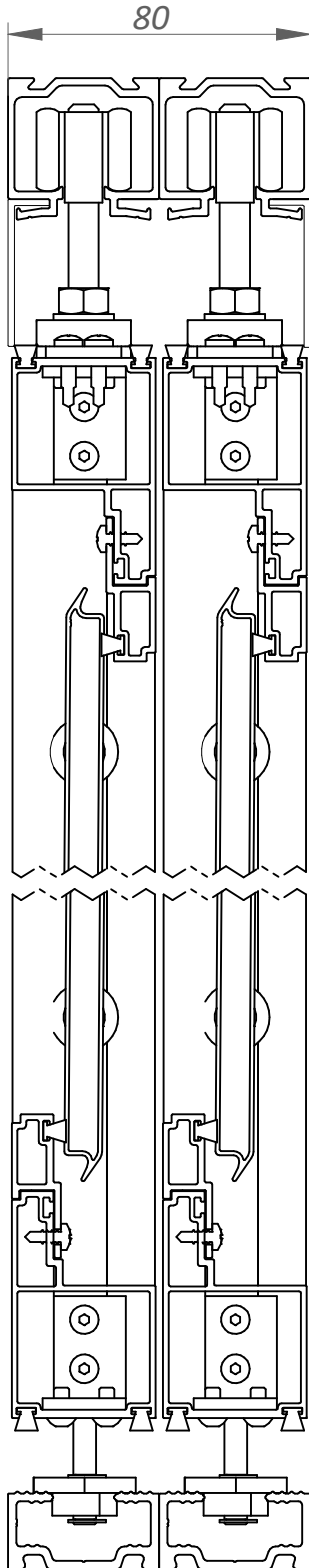
AUFRISS
